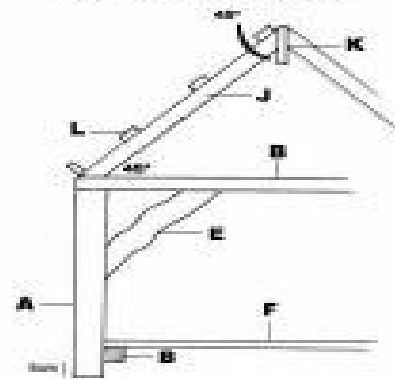
Vooraanzicht kippenhok
